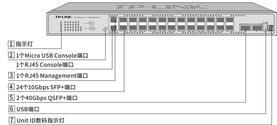
图1-1 TL-NS680-24T2Q前面板示意图
