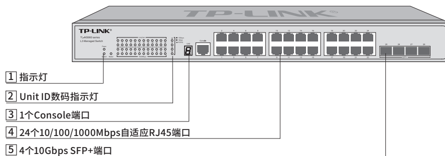
图1-5 TL-NS660-24G4T前面板示意图
