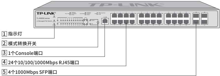
图1-10 TL-NS650-24GP4F前面板示意图
